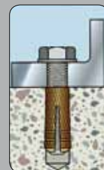
Definitieve bevestiging met metrische schroef of bout.
