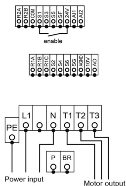
Schaltplan:
