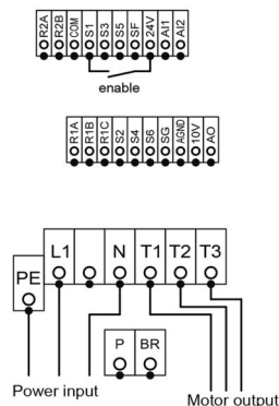
Wiring diagram:
