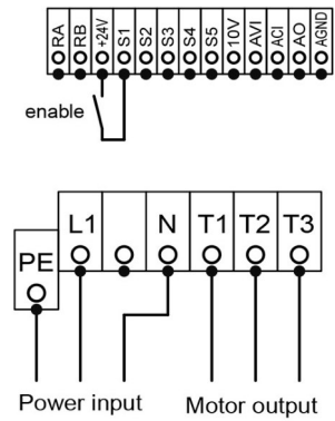
Wiring diagram:
