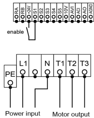
Schaltplan:
