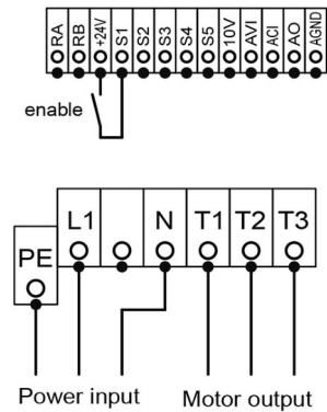
Wiring diagram:
