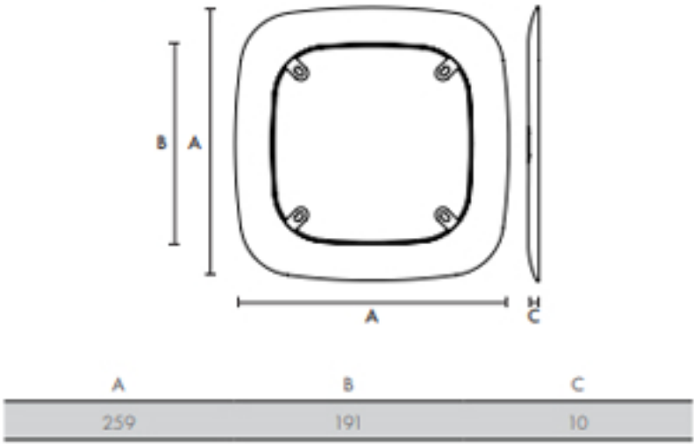
Afmetingen kader (mm)
