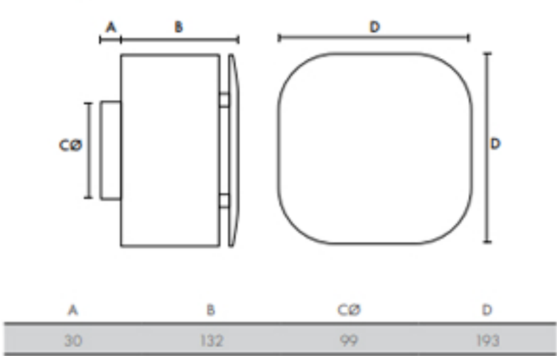
Afmetingen (mm)
